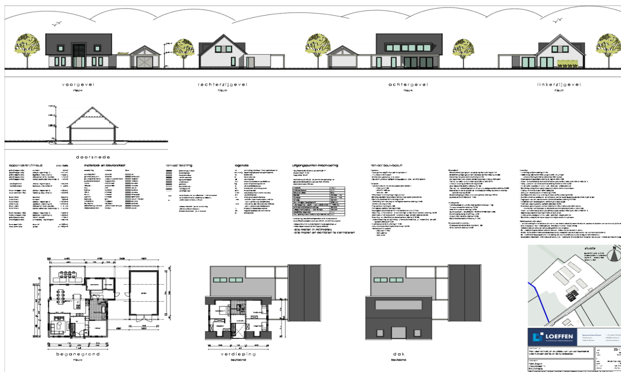
Beoogde situatie. Bron: Loeffen Bouwkundig ingenieursbureau
